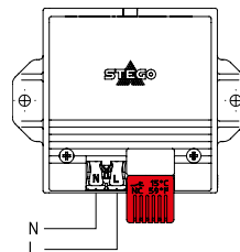
Пример подключения нагревателя с вентилятором CSF 028
