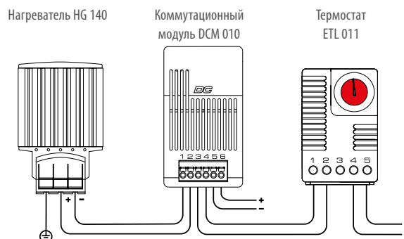
Пример подключения
